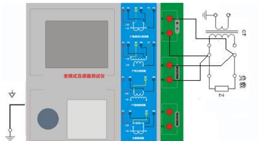
图 2.2 CT 二次负荷试验接线方式
