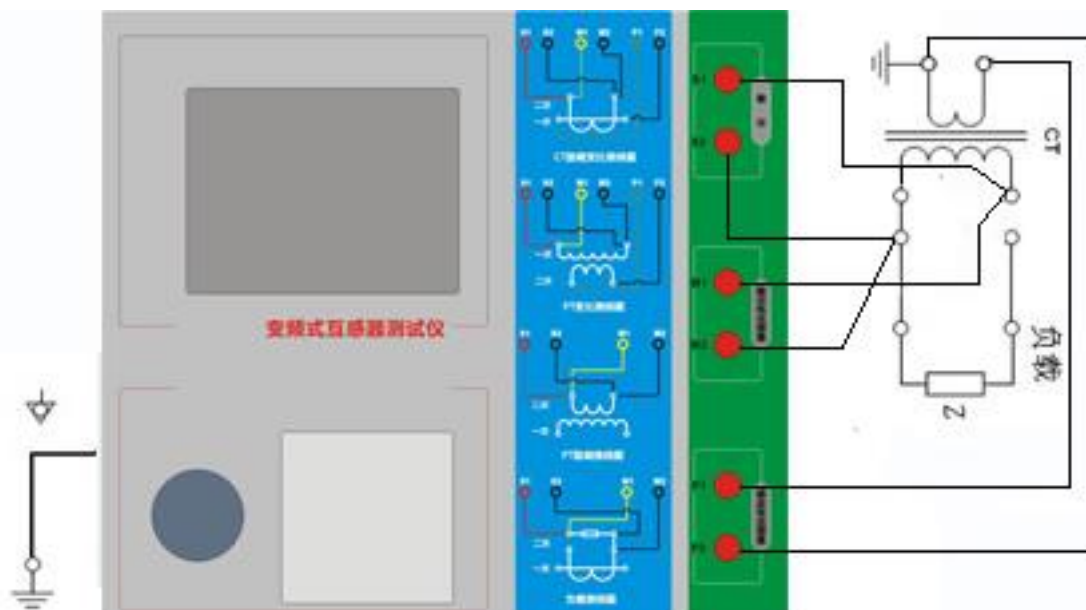
图 2.1 CT 直阻、励磁、变比试验接线方式
