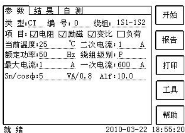
图 2.3 基本参数设置界面
