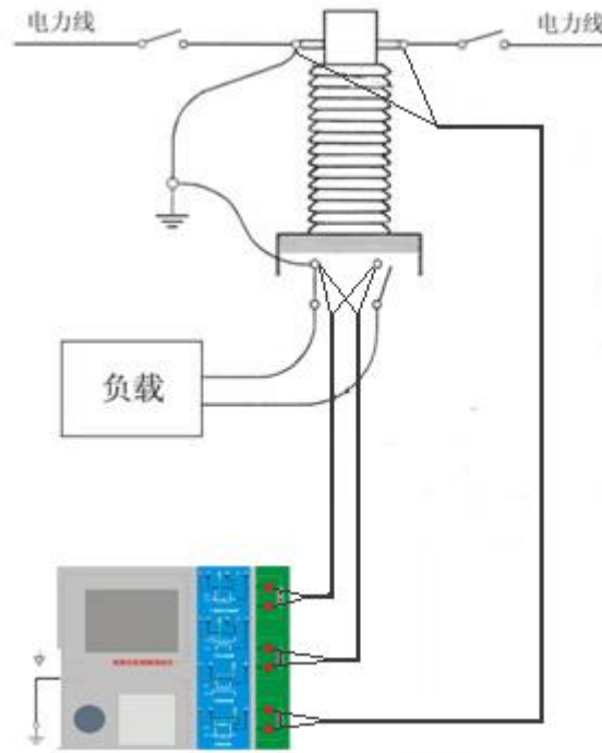
图 C.1 典型接线方式
