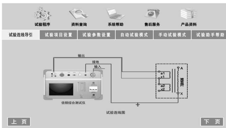
二次绕组加压连线图（无分压器）
