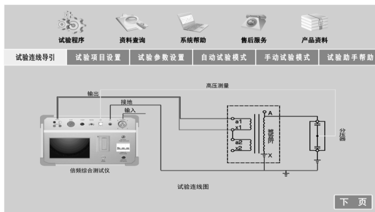
二次绕组加压连线图（有分压器）
