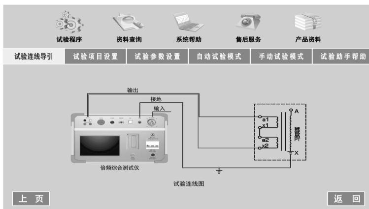
二次绕组串联加压连线图（无分压器）
