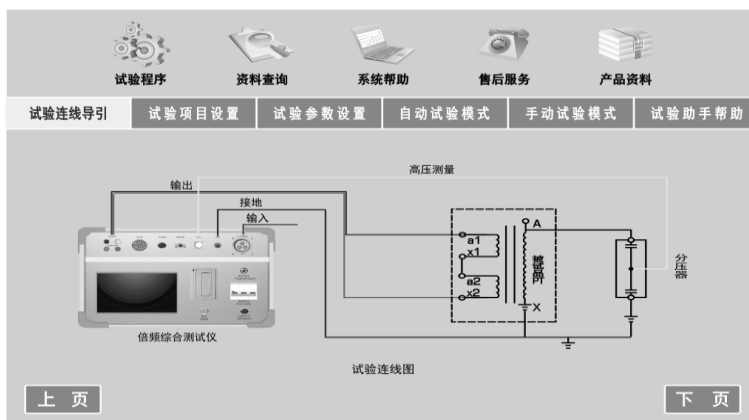
二次绕组串联加压连线图（有分压器）
