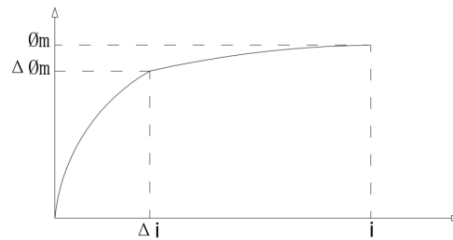
图 1 激励电流与主磁通振幅
